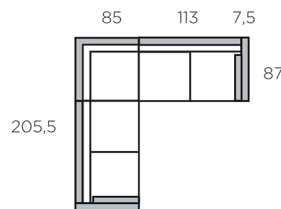
AR5 / 2-wa / 90S / 2-wa / AR5
